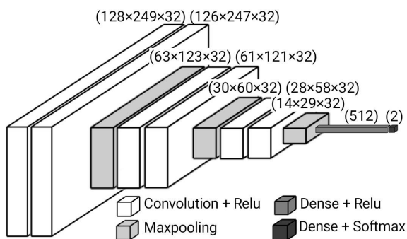
図1 CNNの構造
