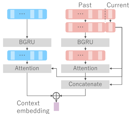
図 4 注意機構付き CMCCE のモデル構造. 青色の図形は韻律埋め込みベクトルを表し, 赤色の図形は文埋め込みベクトルを表す.
