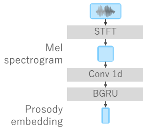
図 3 Prosody Encoder のモデル構造. この図では, ある対話ターンのみにおける韻律埋め込みベクトルの抽出を示している.
