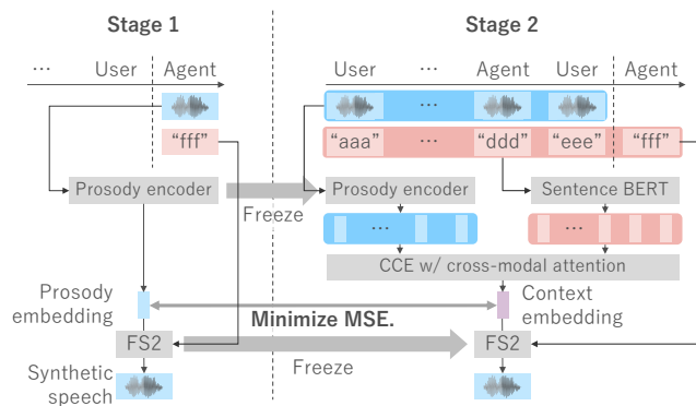
図 5 提案するカリキュラム学習の概念図
