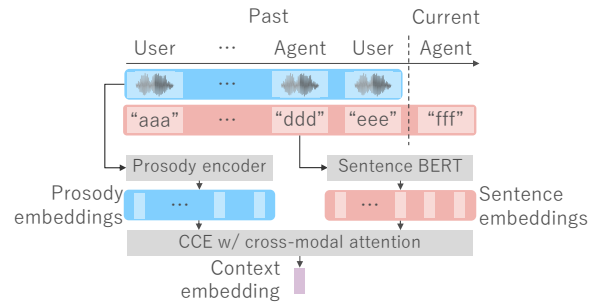
図 2 Cross-Modal CCE (CMCCE) のモデル構造
