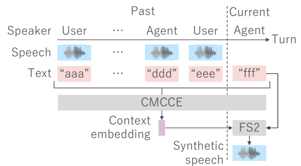
図 1 提案法のアーキテクチャ (“FS2” は FastSpeech2 を意味する)
